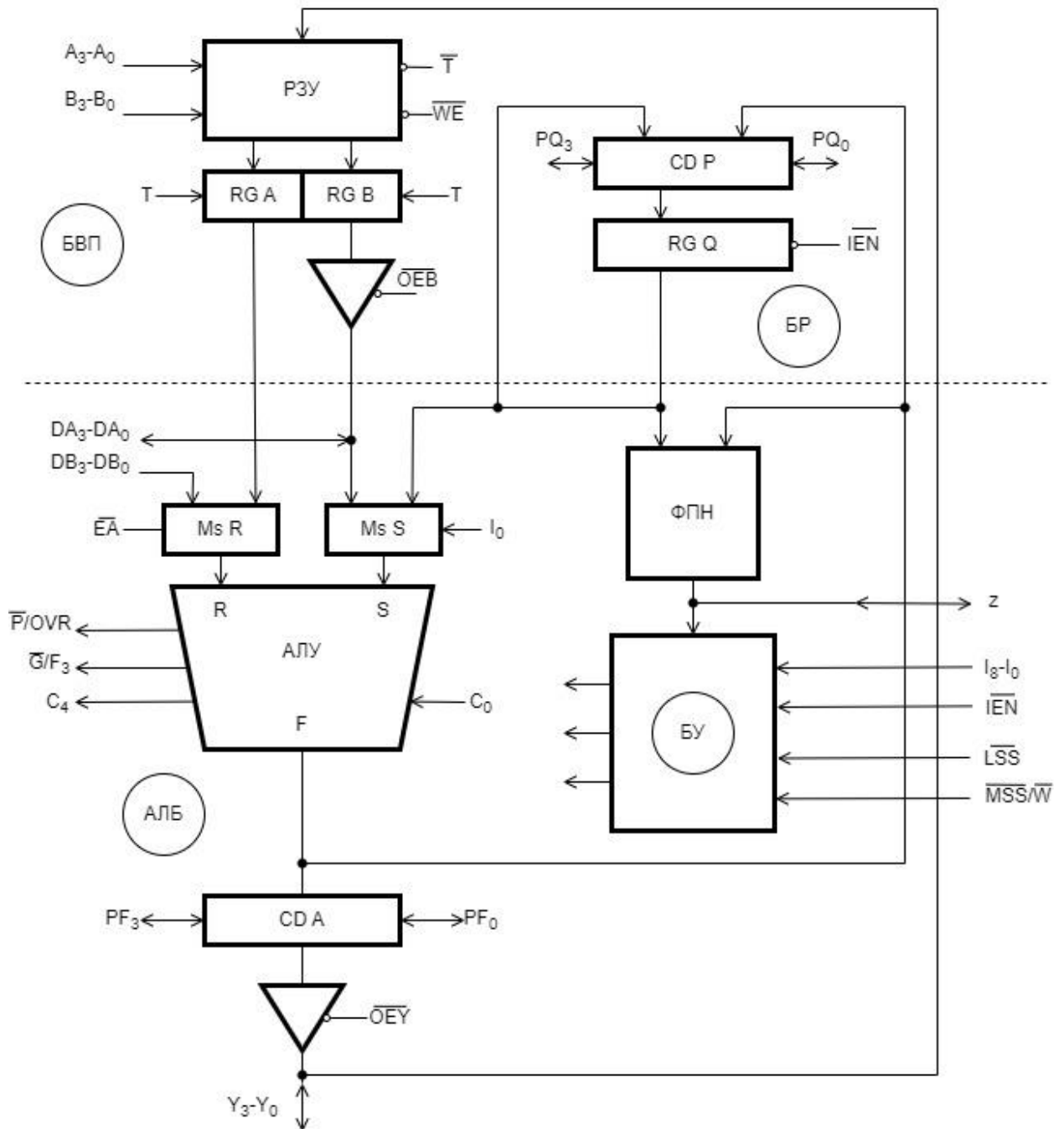
Рисунок 2.1 – Структура K1804BC2
